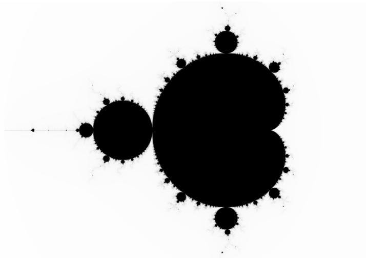
Figur 1: Mandelbrotmængden
